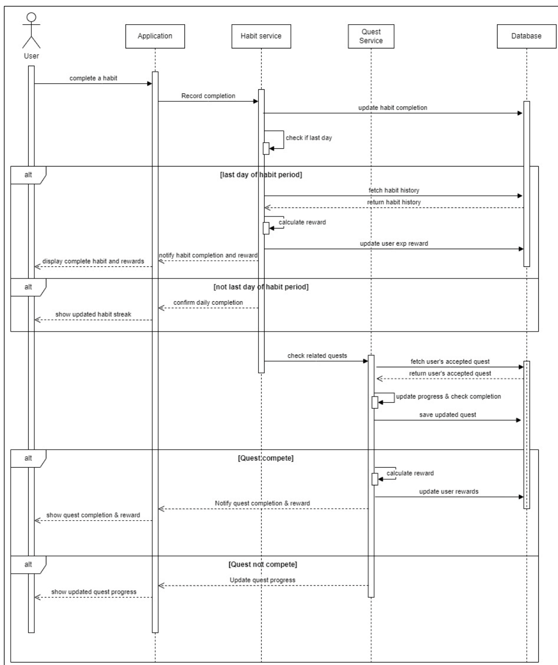
รูป 3.17 Sequence Diagram ระบบภารกิจ
