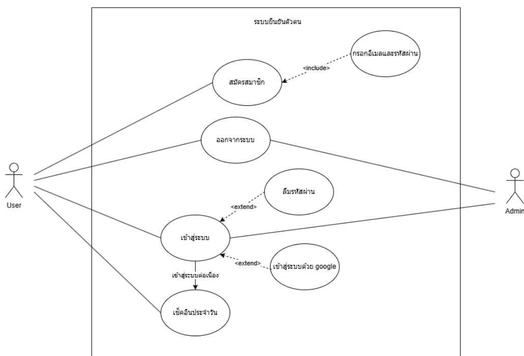
รูป 3.2 Use Case Diagram ของระบบยืนยันตัวตน
