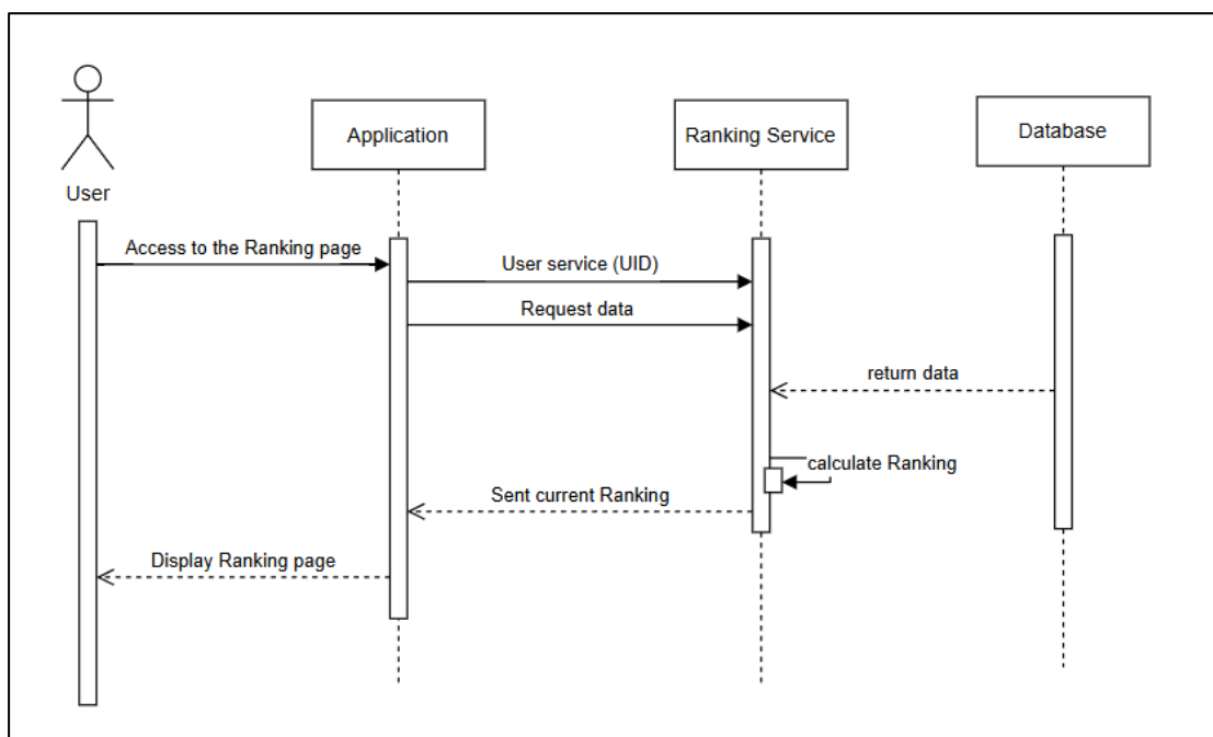
รูป 3.20 Sequence Diagram ระบบกระดานจัดอันดับ
