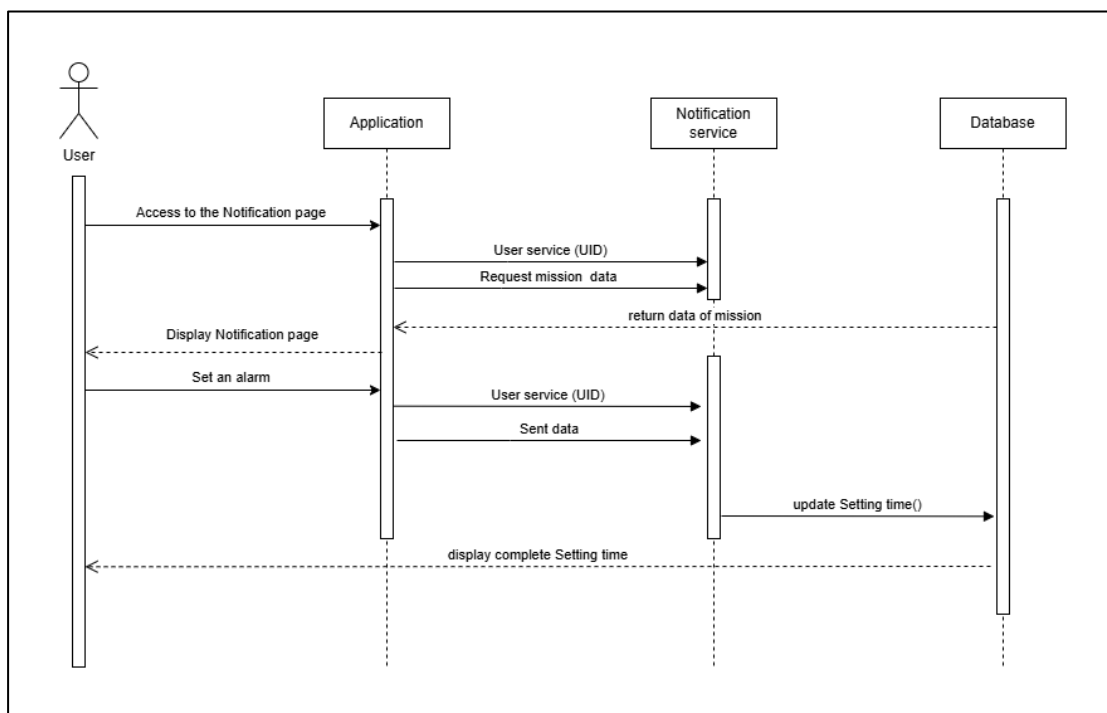
รูป 3.24 Sequence Diagram ระบบแจ้งเตือน
