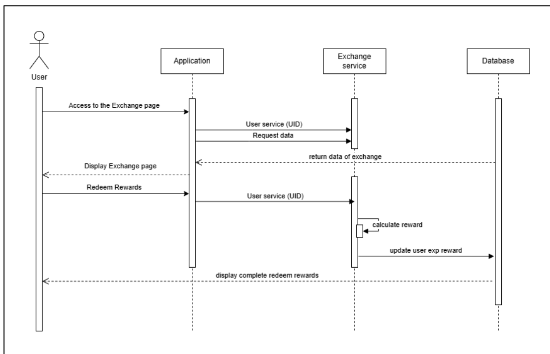
รูป 3.23 Sequence Diagram ระบบแลกรางวัล
