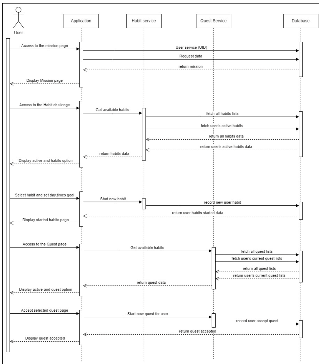
รูป 3.16 Sequence Diagram ระบบภารกิจ
