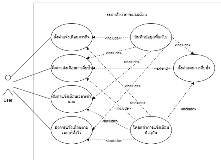
รูป 3.9 Use Case Diagram ของระบบตั้งค่าการแจ้งเตือน
