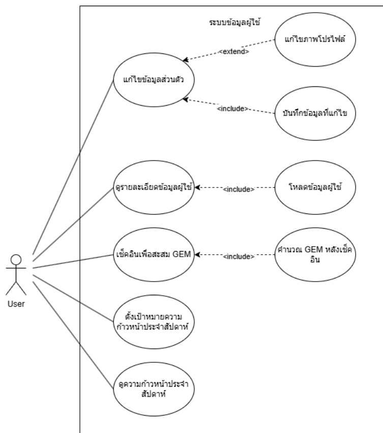
รูป 3.4 Use Case Diagram ของระบบแก้ไขข้อมูลผู้ใช้
