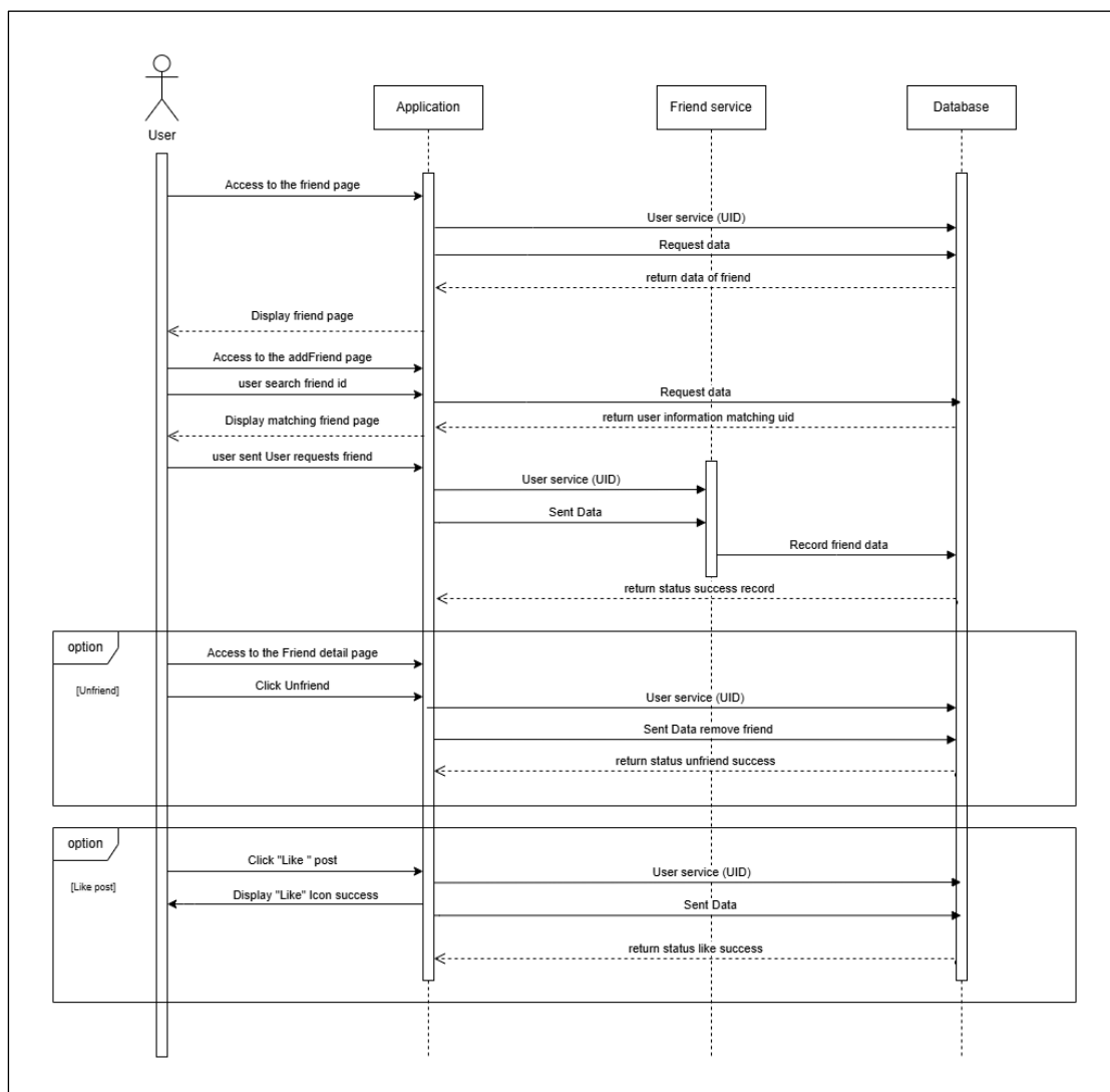
รูป 3.21 Sequence Diagram ระบบเพื่อน
