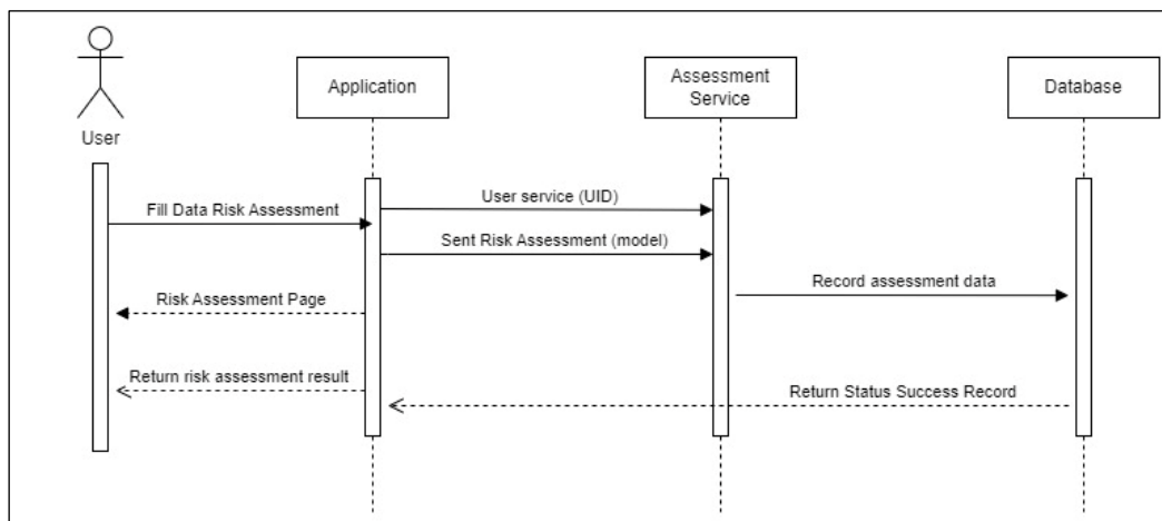
รูป 3.14 Sequence Diagram ระบบประเมินสุขภาพ
