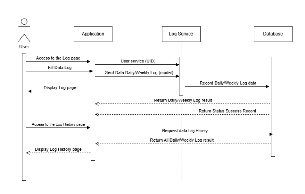
รูป 3.15 Sequence Diagram ระบบบันทึกสุขภาพ
