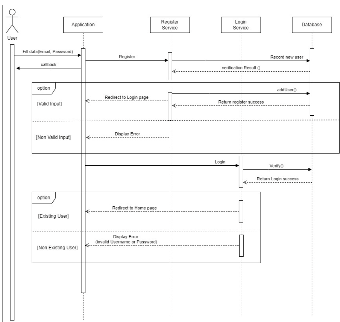
รูป 3.12 Sequence Diagram ระบบลงทะเบียน
