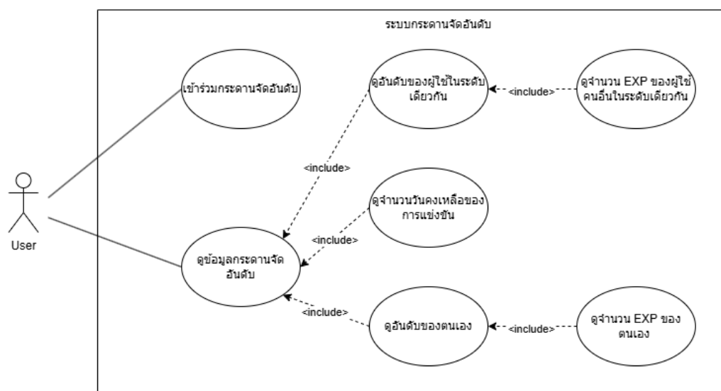
รูป 3.7 Use Case Diagram ของระบบกระดานจัดอันดับ
